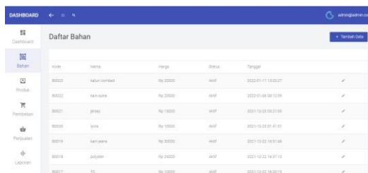
Gambar 13 Halaman Bahan
