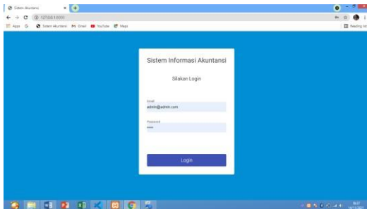
Gambar 11 Halaman Login
