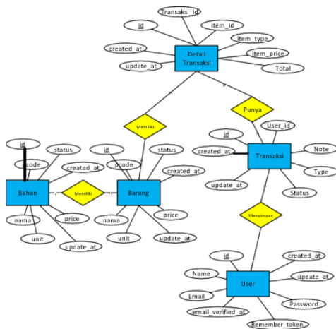
Gambar 5. Entity Relationship Diagram Sistem yang diusulkan
