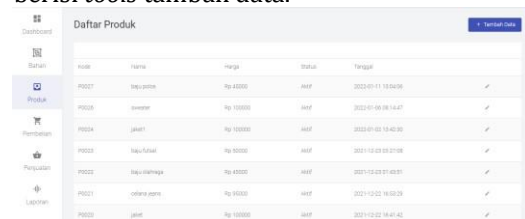
Gambar 16 Halaman Produk
