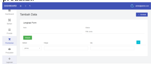
Gambar 19 Halaman Pembelian
