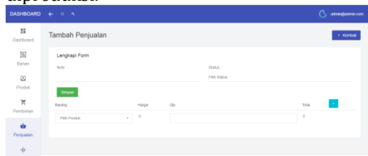
Gambar 20 Halaman Penjualan
